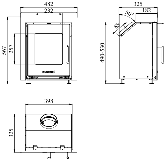
Morsø S81
