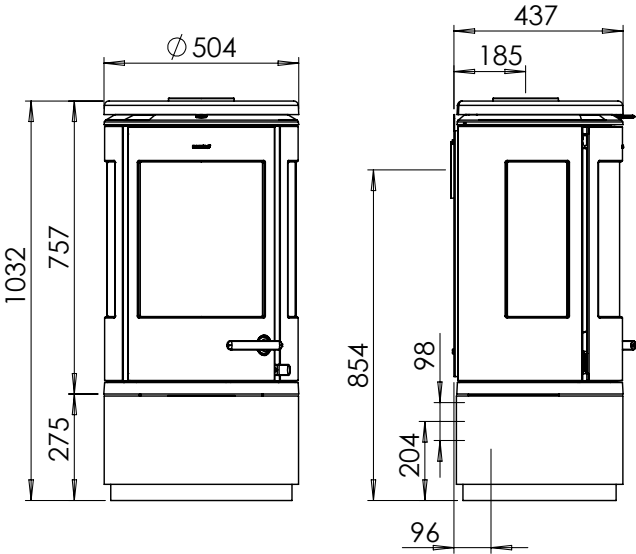
Morsø 7940
