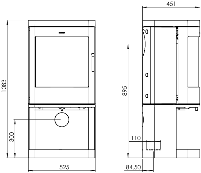
Morsø 8643
