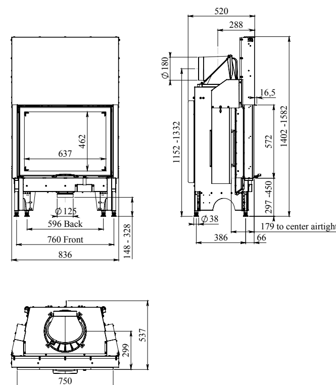
Morsø S101-12
