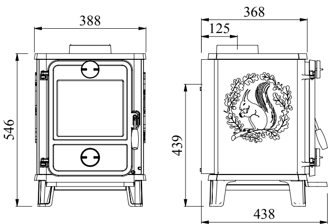
Morsø 1412
