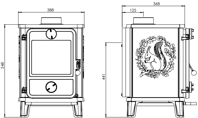
Morsø 1010
